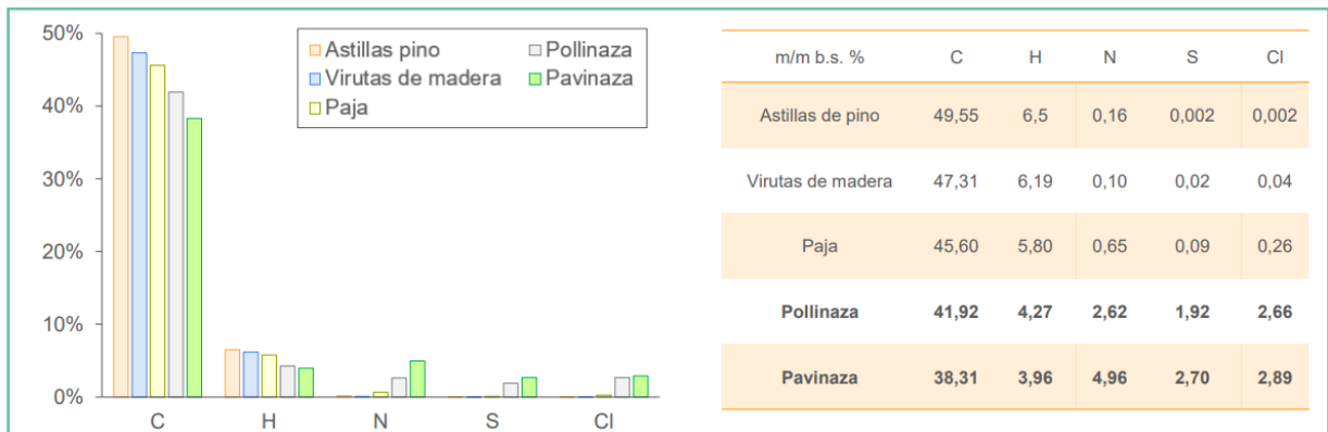
Gráfica y tabla comparativa del análisis elemental de los distintos materiales.
